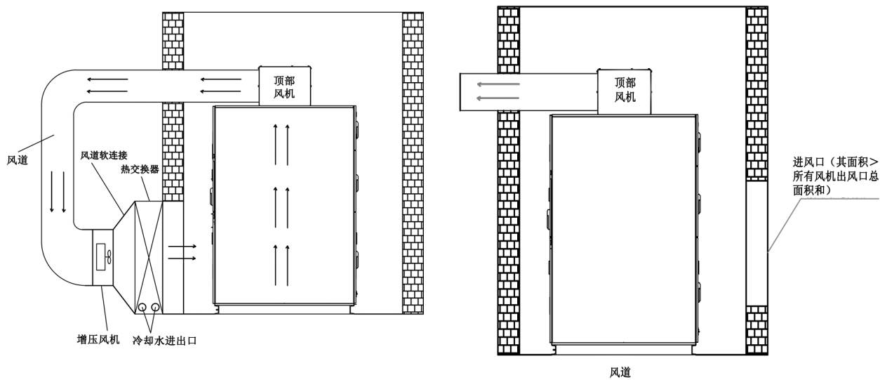
图7.5 空水冷图
