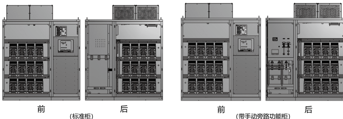
图3.20 10kV单元柜柜布置图
