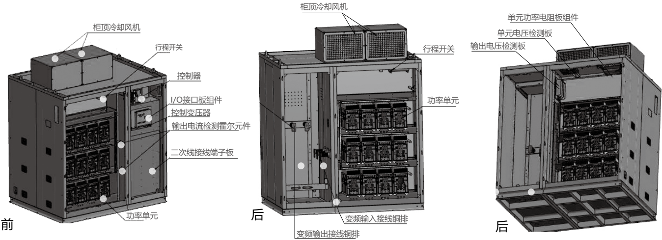
图3.18 典型单元柜排布图
