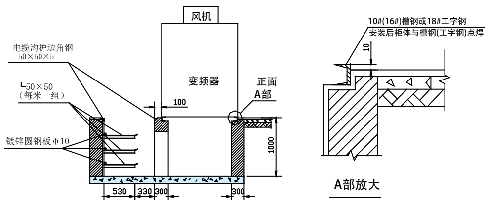
图7.6 电缆沟
