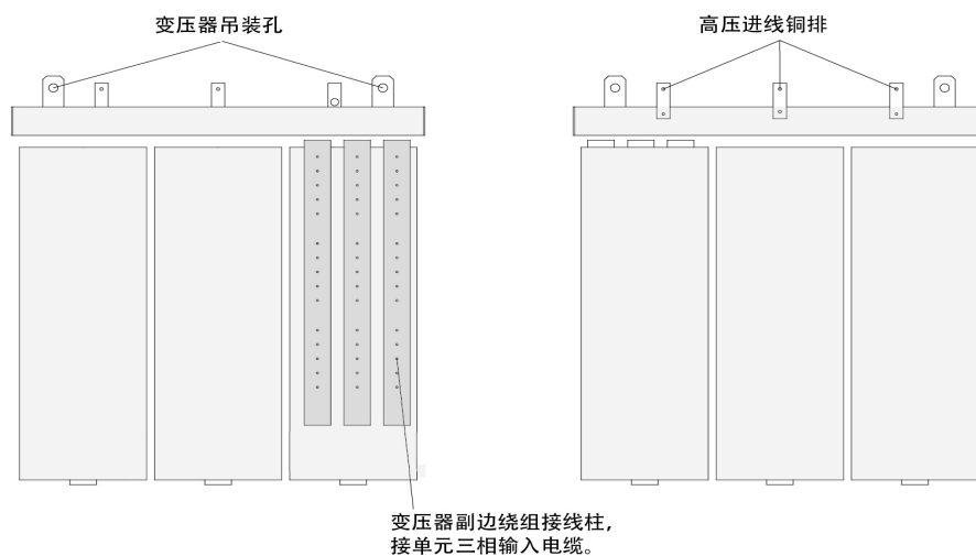
图3.16 变压器吊装孔示意图
