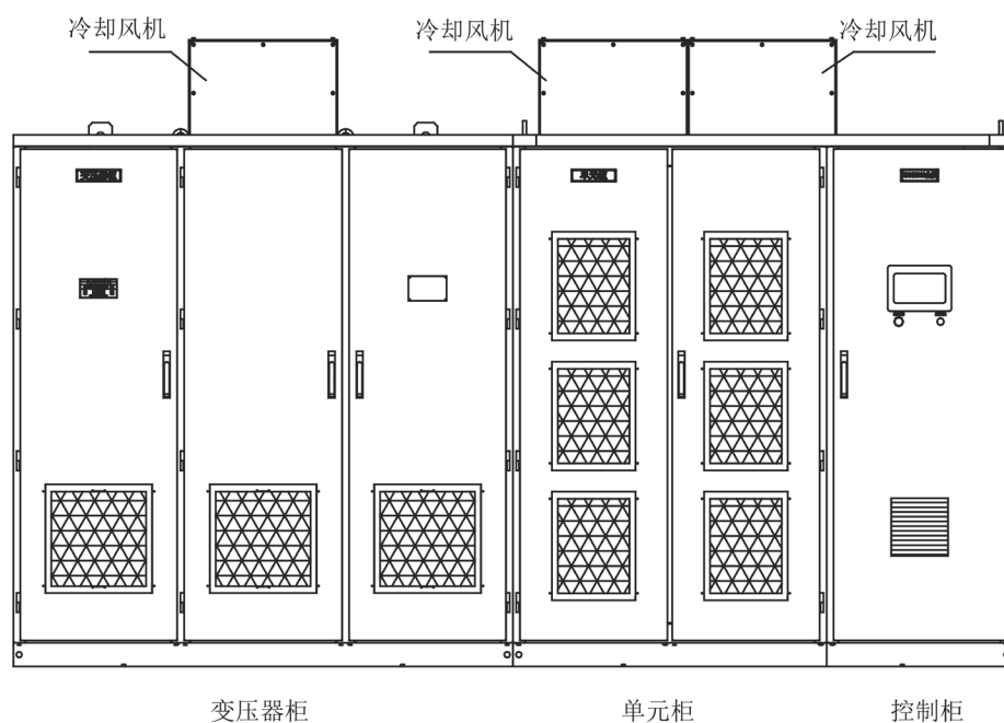
图3.14 变频器典型柜体
