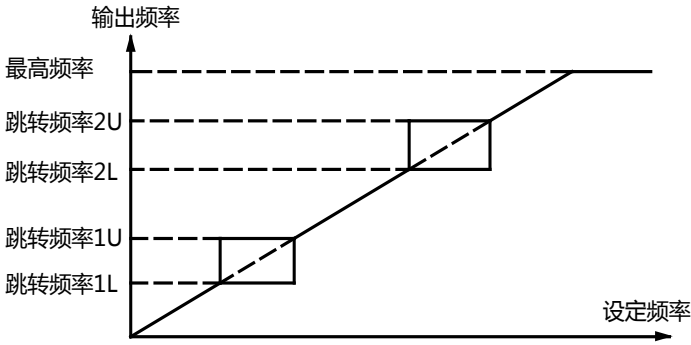
图5.24 跳转频率
