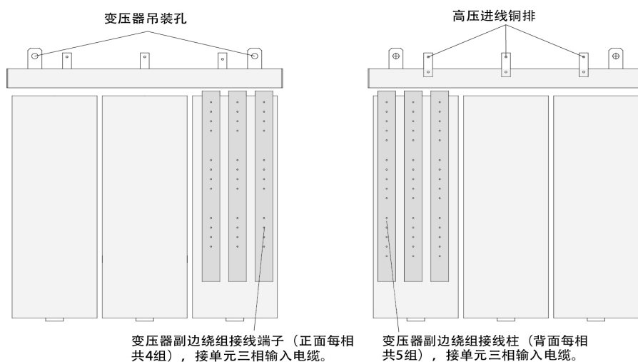
图3.17 变压器副边结构图
