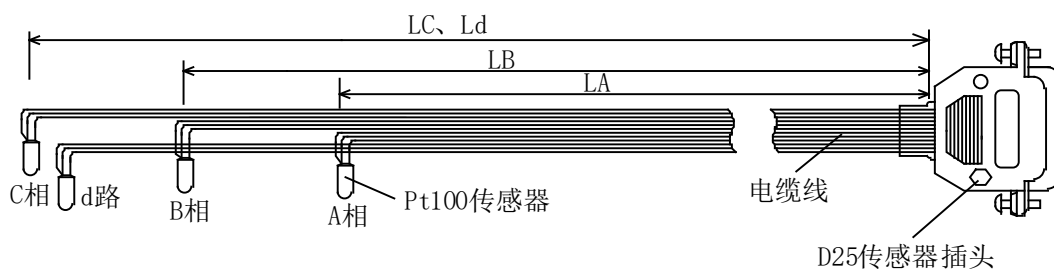
G/I型四路电缆连接示意图
