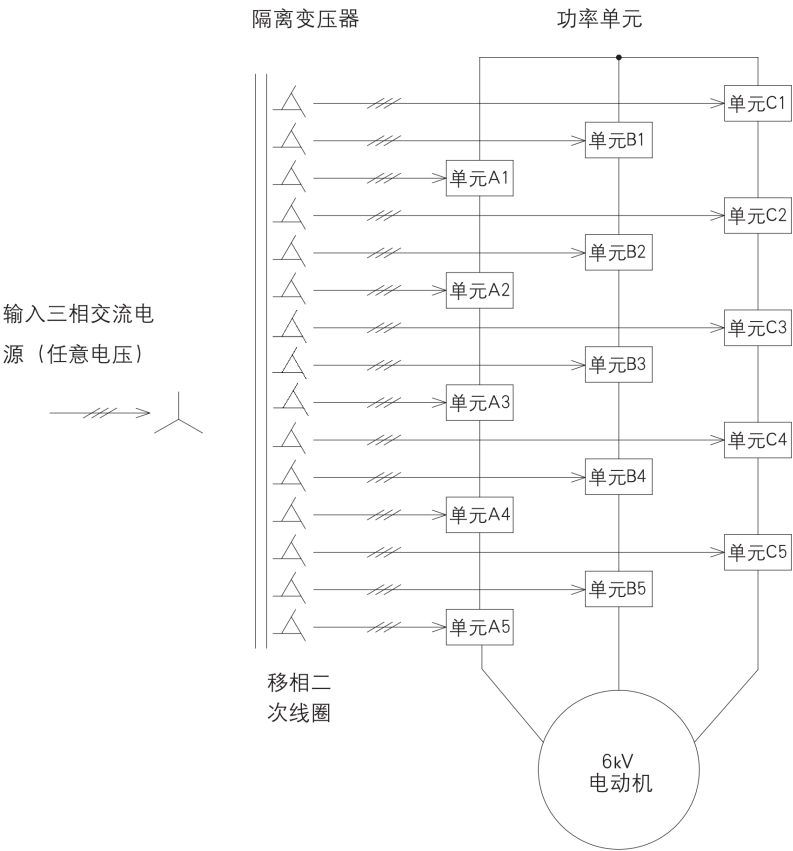
图3.2 变频器主回路图（6kV为例）
