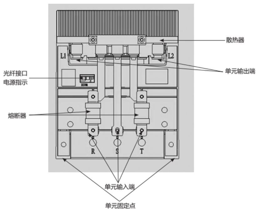
图3.12 功率单元外形图
