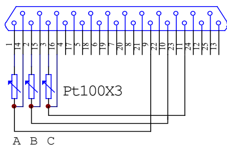
D/E/F型三路插头内部示意图
