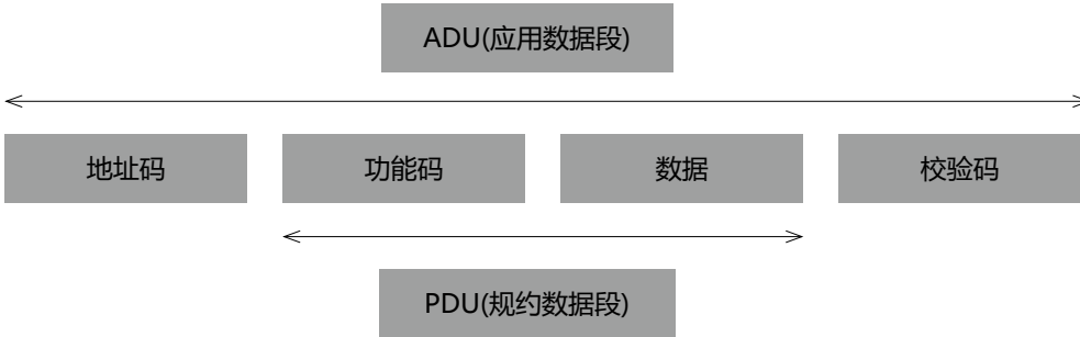
图11.2 数据包结构
