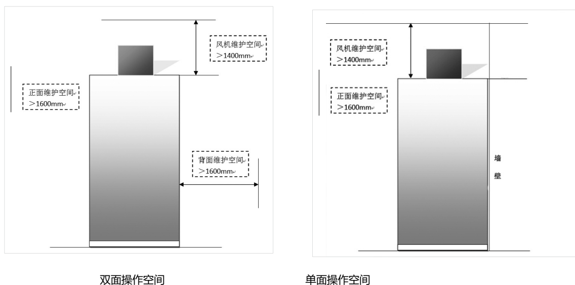
图7.2 柜体摆放空间
