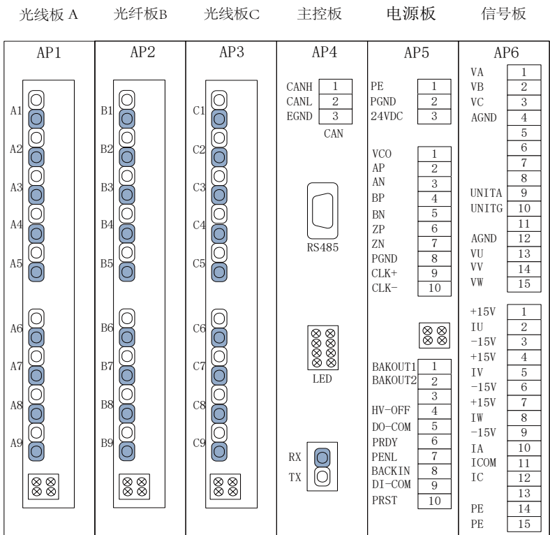
图3.6 控制器面板示意图
