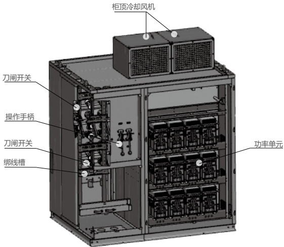
图3.19 带手动旁路柜外形图
