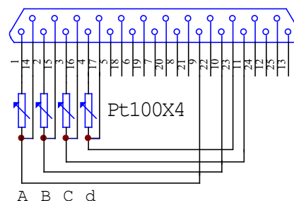
G/I型四路插头内部示意图
