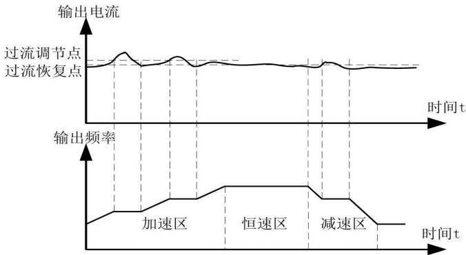
图6.3 过流调节示意图
