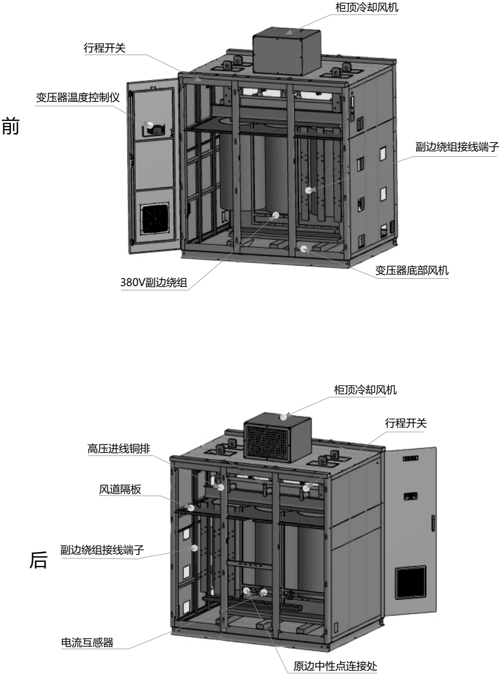
图3.15 典型变压器柜装配图
