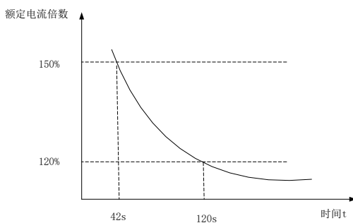
图6.2 反时限保护示意图
